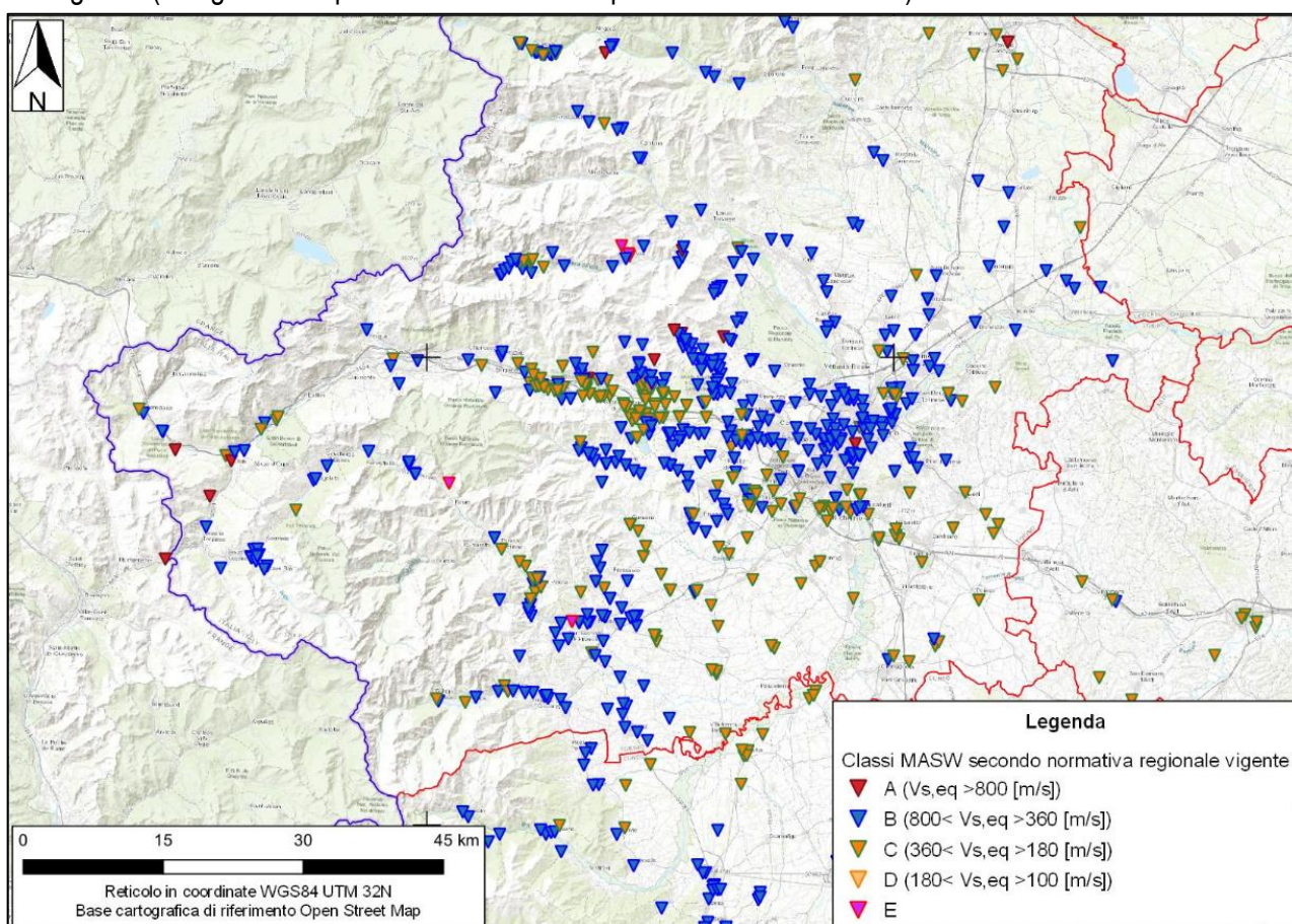
Distribuzione V_{s,eq} nella provincia di Torino. Database Techgea
